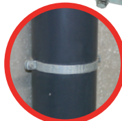
ABRACADEIRA DE ESPÍGÃO COM PARAFUSO SOLDADO Drain pipe clamp with welded screw / Colliers à pointe a/ vis soudée / Abrazadera de Espigón c/ Tornillo Soldado
